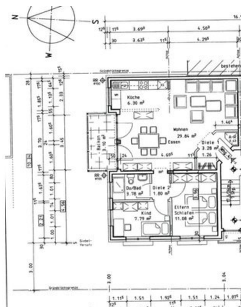
Grundriss
